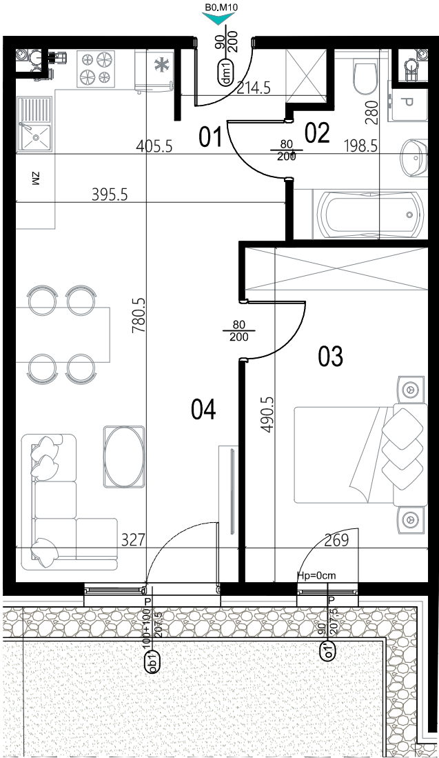
Rzut lokalu mieszkalnego 0m 1m 2m 3m
