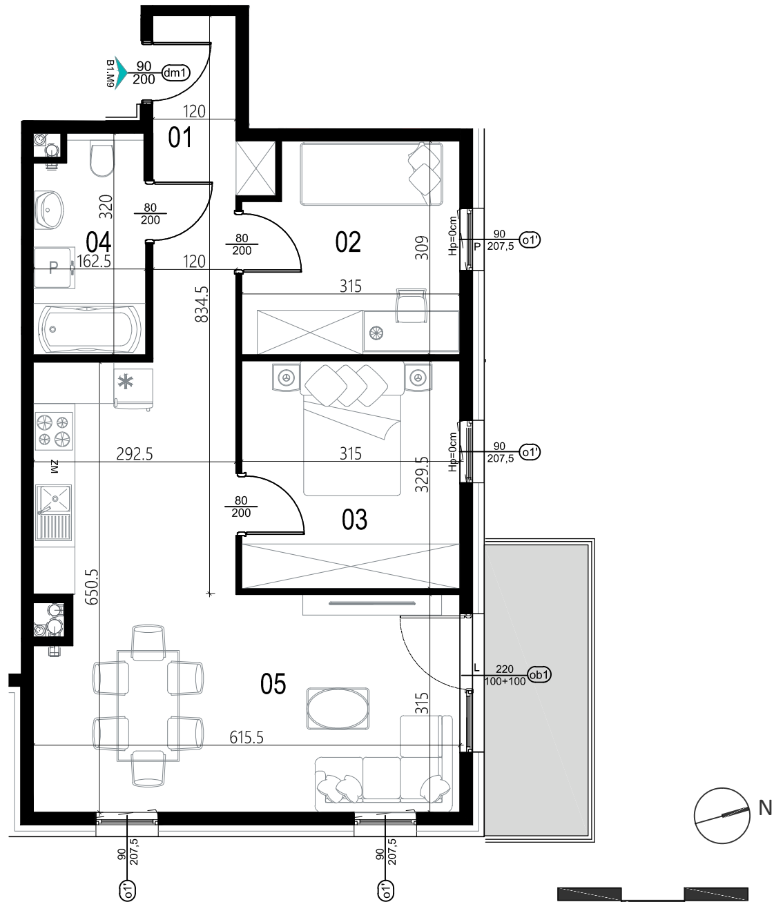
Rzut lokalu mieszkalnego
