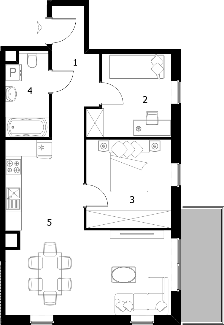
Rzut lokalu mieszkalnego
