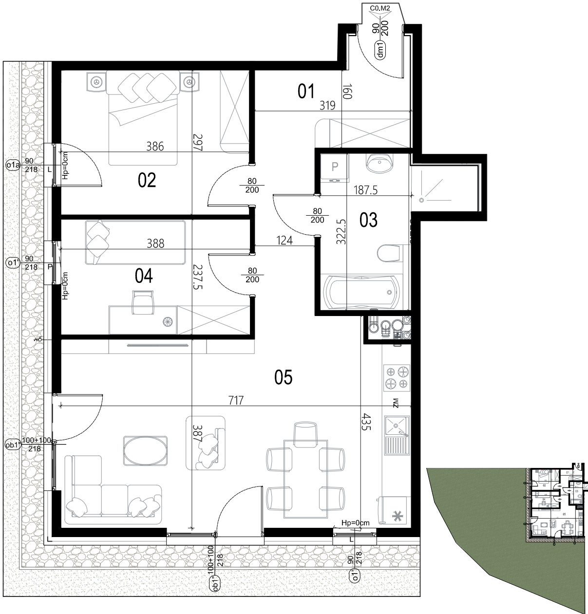
Rzut lokalu mieszkalnego
