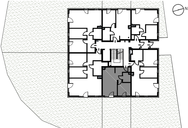
Rzut kondygnacji - parter
