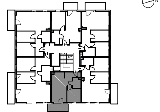
Rzut kondygnacji - I piętro
