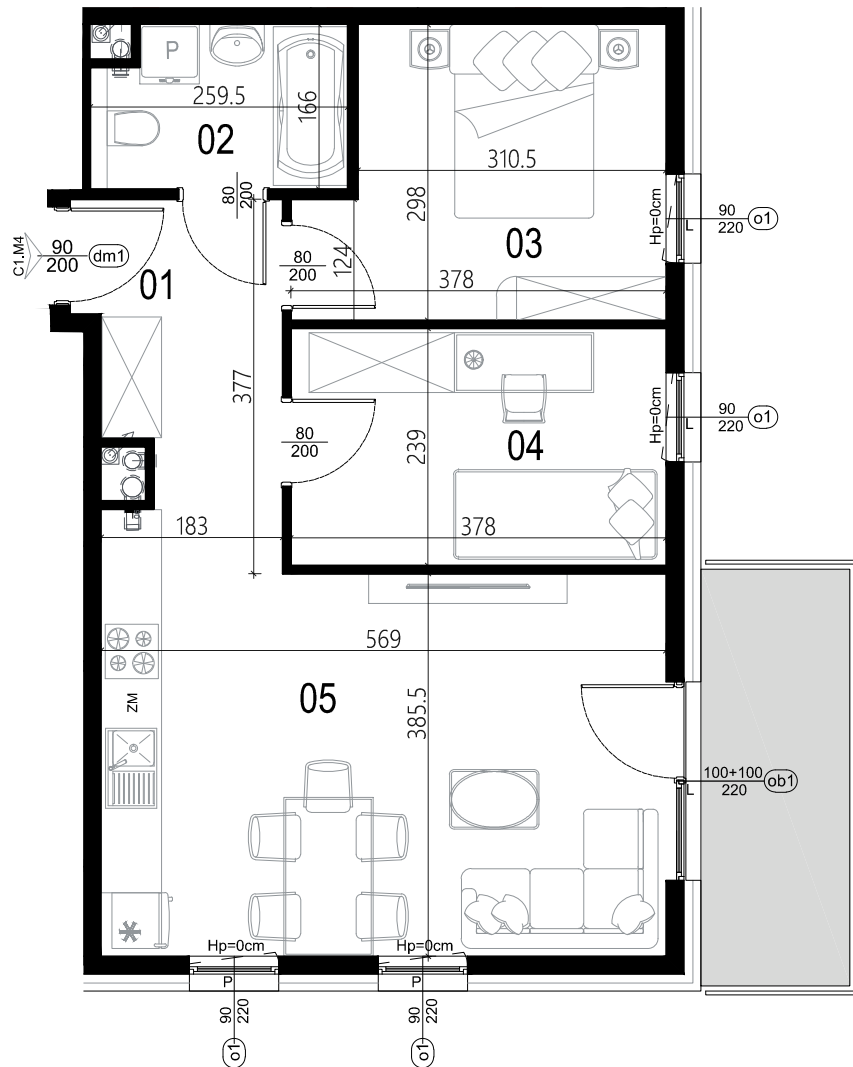
Rzut lokalu mieszkalnego
