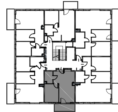
Rzut kondygnacji - I piętro
