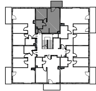
Rzut kondygnacji - II piętro
