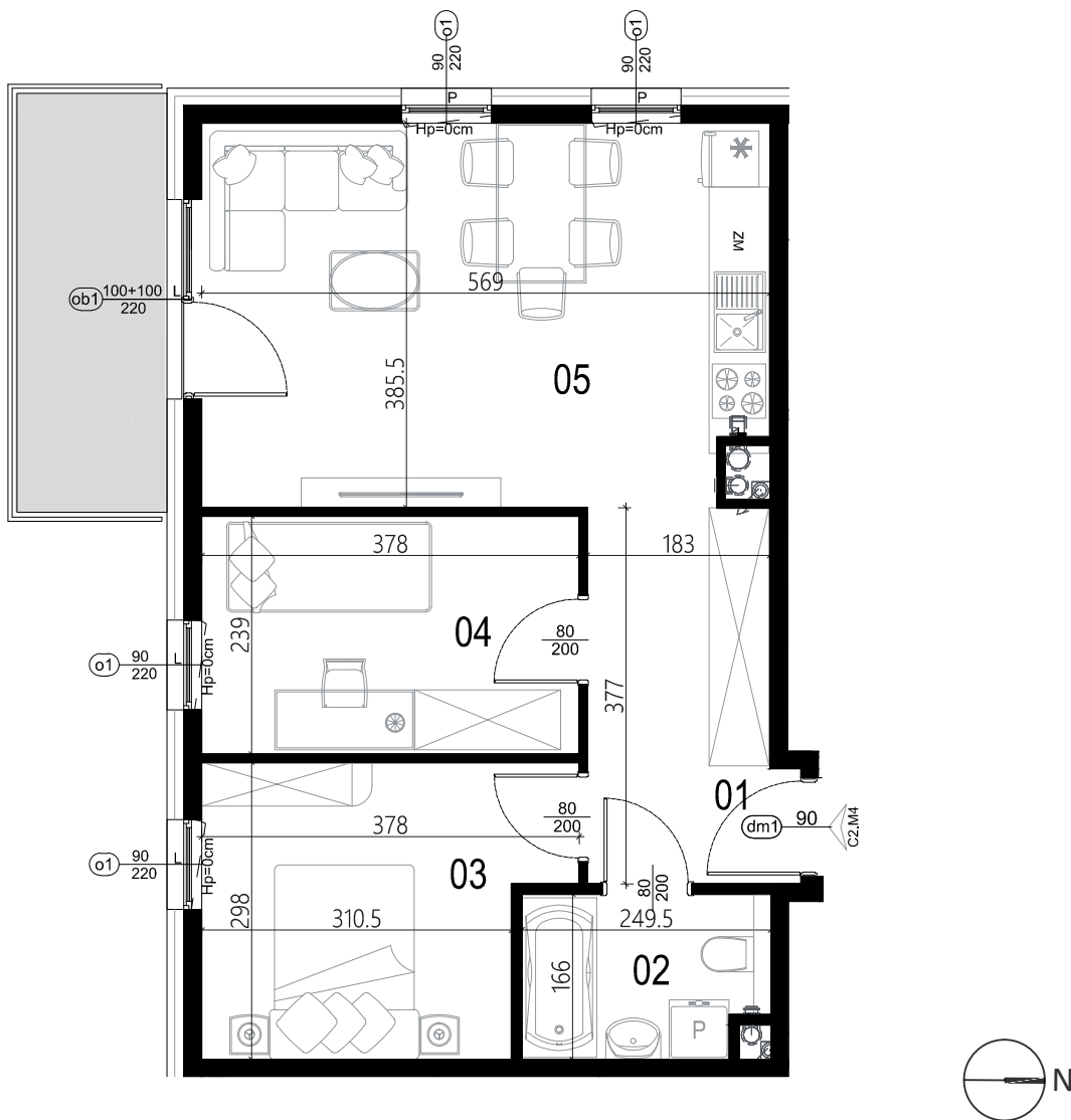
Rzut lokalu mieszkalnego
