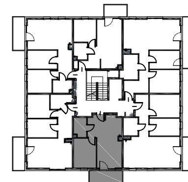
Rzut kondygnacji - II piętro
