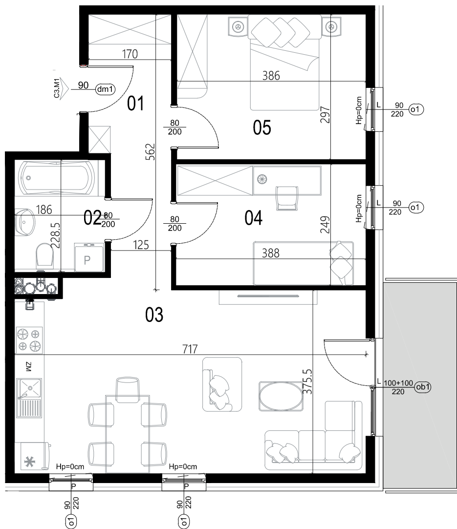
Rzut lokalu mieszkalnego
