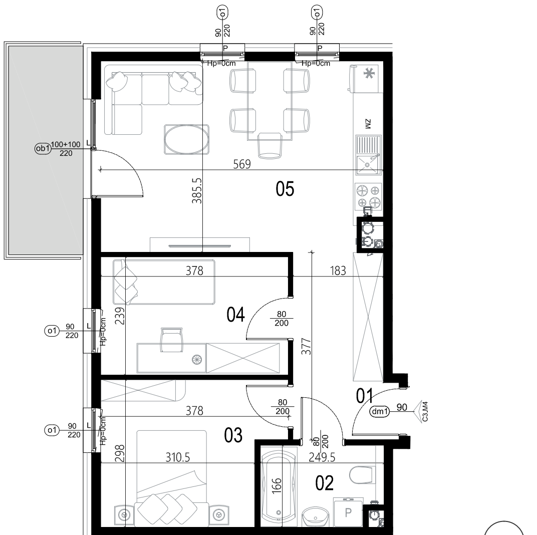
Rzut lokalu mieszkalnego
