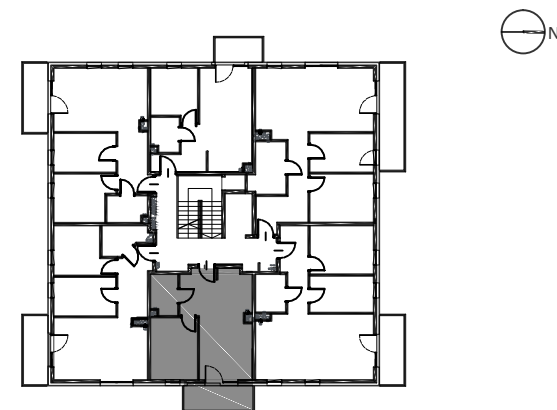
Rzut kondygnacji - III piętro
