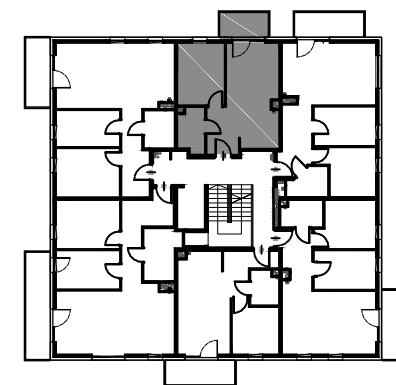
Rzut kondygnacji - III piętro
