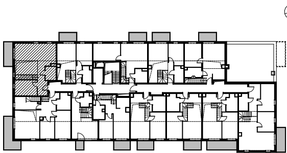
B4.03 82,70m 2 Budynek B1 IV Piętro z antresolą
