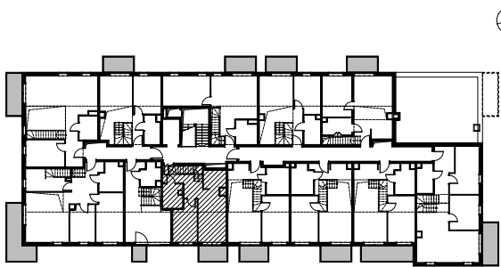
B4.13 62,45m 2 Budynek B1 IV Piętro z antresolą
