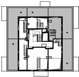
Rzut kondygnacji z lokalizacją mieszkania - antresola
