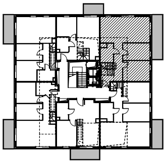
Rzut kondygnacji z lokalizacją mieszkania - IV piętro
