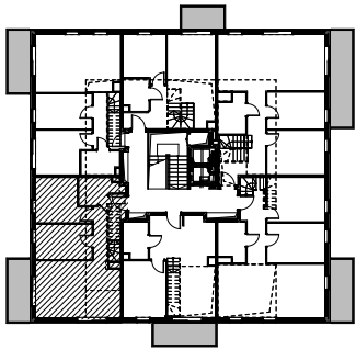
Rzut kondygnacji z lokalizacją mieszkania - IV piętro
