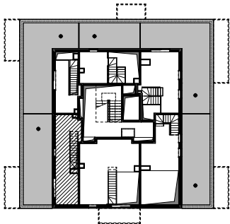
Rzut kondygnacji z lokalizacją mieszkania - antresola
